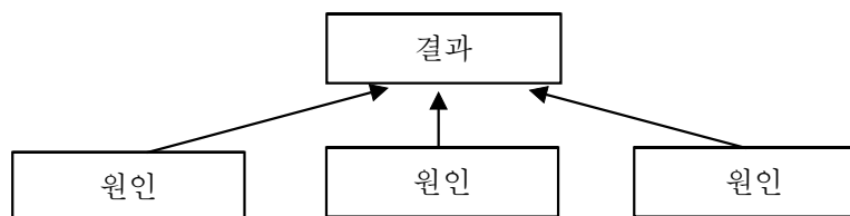
(원인-결과 구조)
